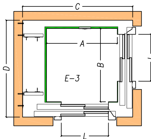
Ascensore elettrico - - Dimensioni europee Electrical lift - - European dimensions
